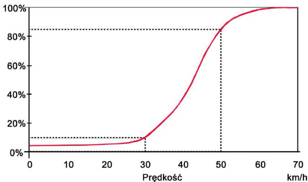
Wykres 1.2. Zależność między prędkością pojazdu a prawdopodobieństwem śmierci pieszego [11]
